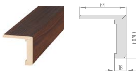
UHOLNÍK S PREDĹŽENÝM PEROM PRE NASTAVITELNÉ ZÁRUBNE
